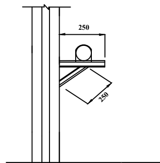
Giá đỡ đường ống DN100
