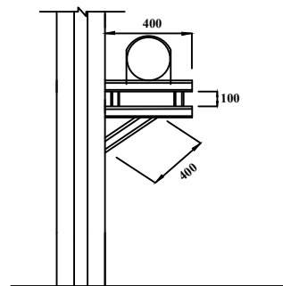
Giá đỡ đường ống DN200
